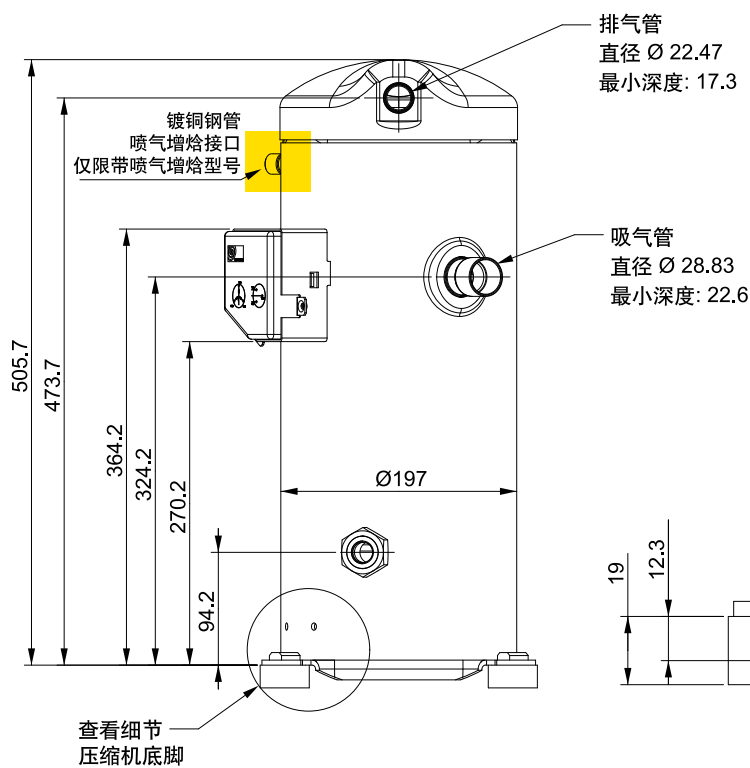
压缩机底脚细节
