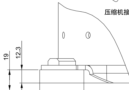
压缩机底脚细节
