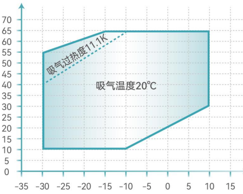
YM34E2G ~ YM410E1G 适用此运行范围图
