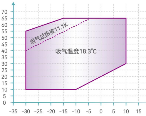
YM560E1G-100适用此运行范围图
