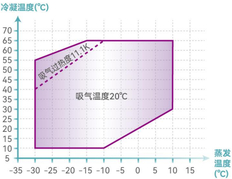
YM34E1G ~ YM240E1G 适用此运行范围图
